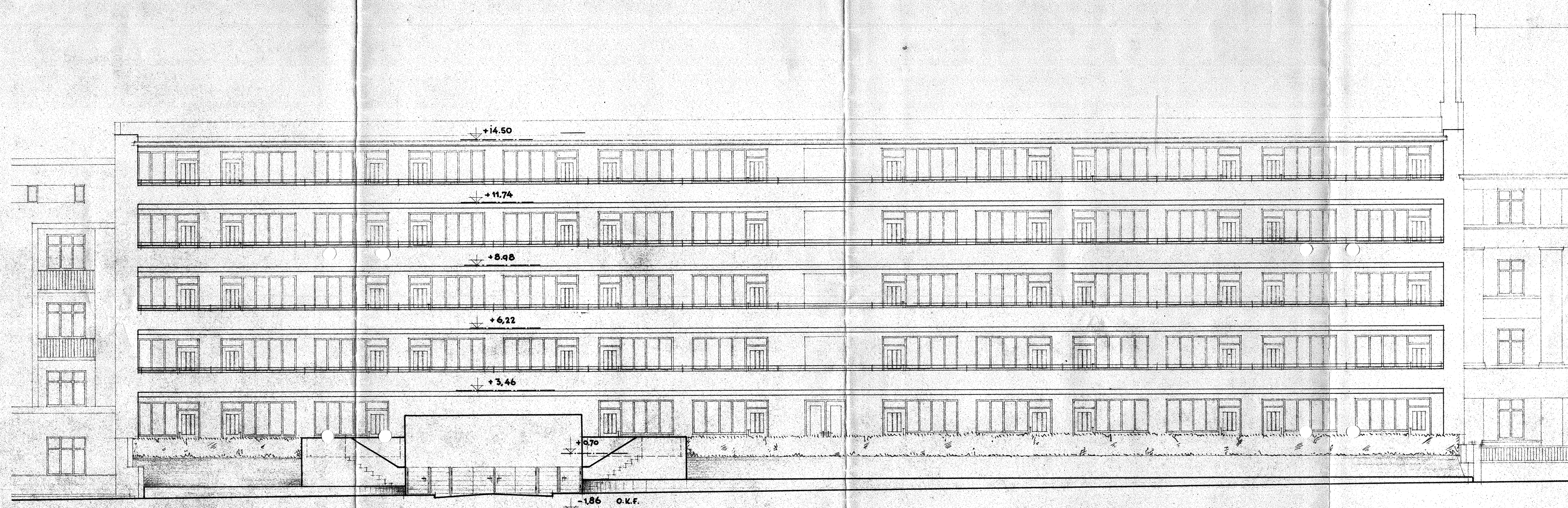
ANSICHT SCHWALBENPLATZ :
